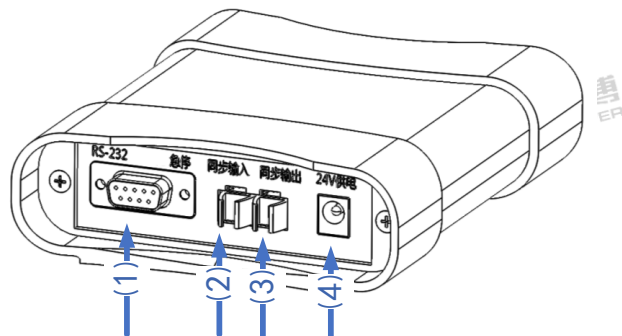
图 95 触发终端后面板功能划分
