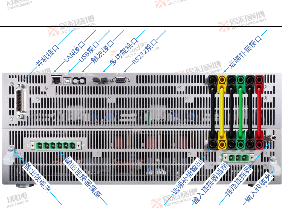
图 23 后面板接口说明图
