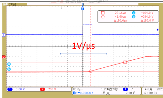
图 57 输出摆率示例
