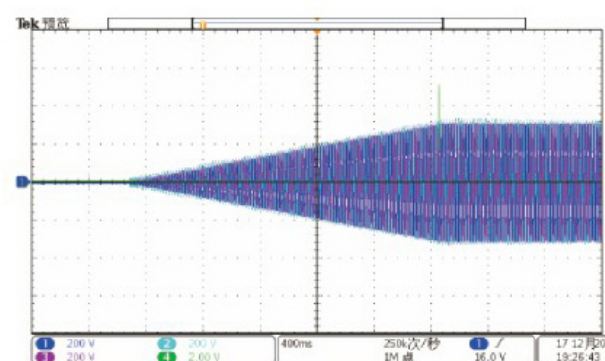
缓启动波形
