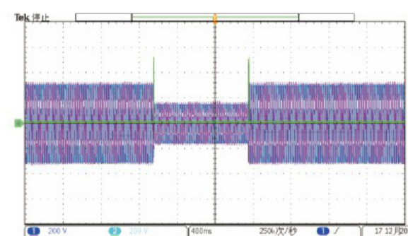
电压突变
