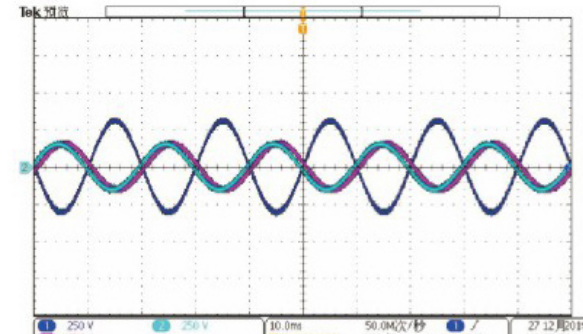
三相不平衡
