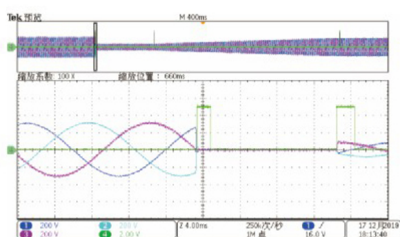
60°低电压穿越
