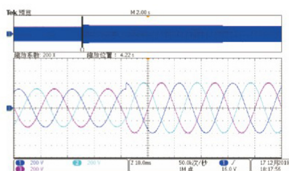
90°高电压穿越
