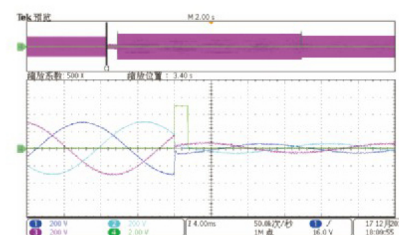
270°高低电压穿越联合测试
