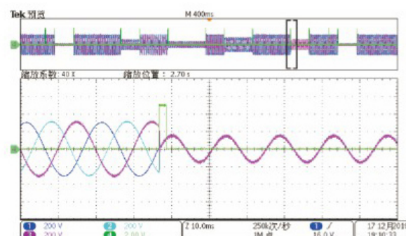
电压相位变化
