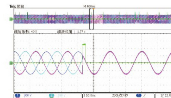
相位扰动
