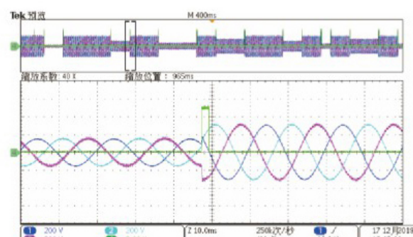
电压扰动
