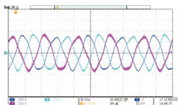
间谐波叠加波形
